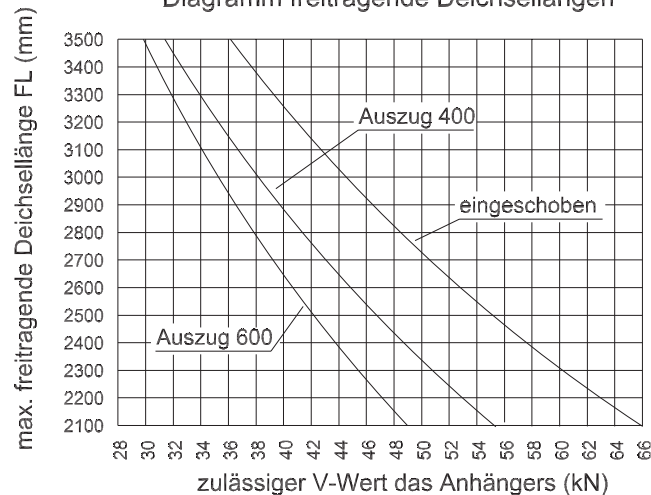
Diagramm freitragende Deichsellängen
