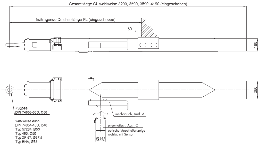
Diagramm freitragende Deichsellängen
